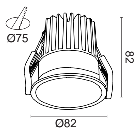
R12
