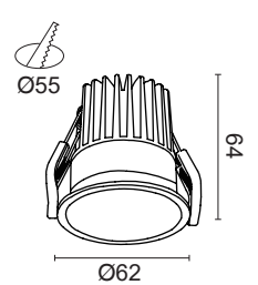
R6
